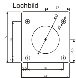
Bohrschablone für Stahleinbaufansch und/oder Schutzkappe im Lieferumfang
